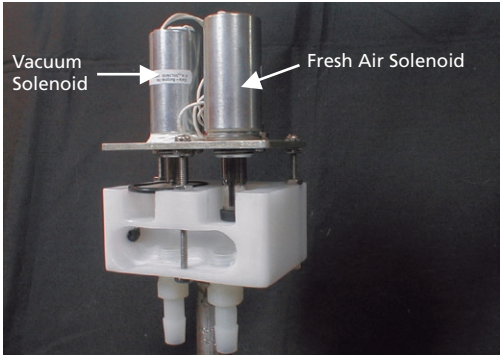
CoPulsation werkt met twee kleppen. De ene zorgt voor vacuüm in de pulsatieruimte en de andere voor atmosferische lucht. De beide kleppen worden om en om geopend, waarbij er dertig milliseconden zit tussen het sluiten van de ene en het opengaan van de andere. Zo kunnen de lucht en het vacuüm niet vermengd worden.
