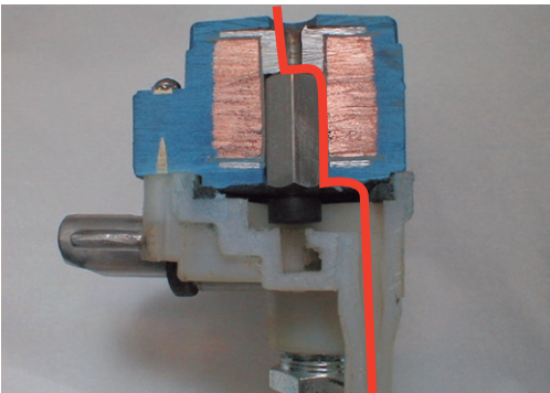
Bij een gangbaar systeem laat een zuiger zowel lucht als vacuüm de pulsator binnen. De zuiger gaat op en neer, waarbij er tijdens de beweging van de zuiger een open verbinding is tussen het vacuüm en de atmosferische lucht. De luchtinlaat is daardoor noodgedwongen klein en het resultaat is een inefficiënte werking van de pulsator.
